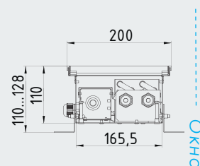
Разрез
