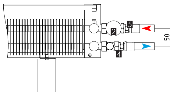
Подключение сбоку
