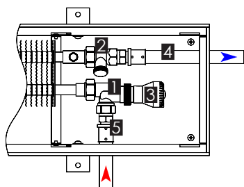
Разностороннее подключение
