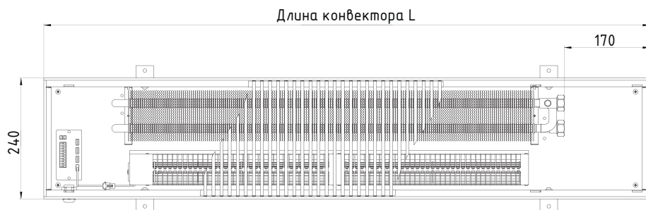
Вид сверху
