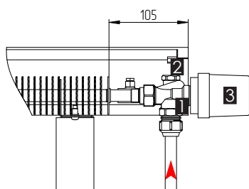
Подключение снизу
