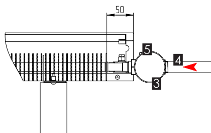
Подключение сбоку
