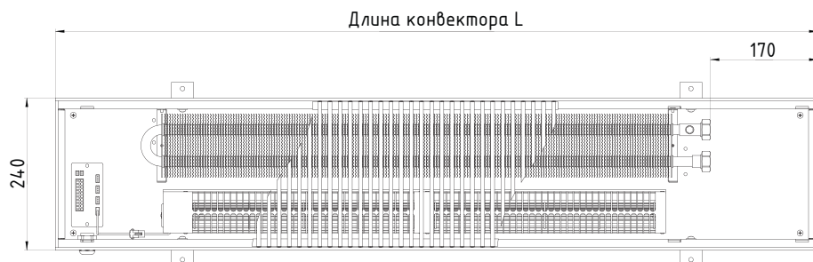
Вид сверху
