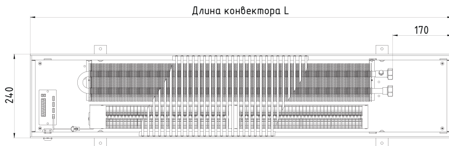
Вид сверху
