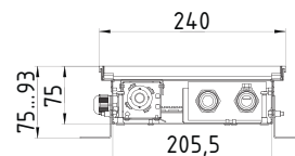
Разрез
