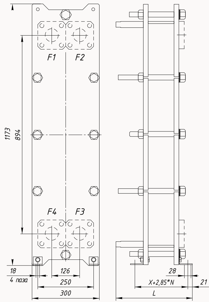
I LP-50L (Расчетное давление 1,0 Мпа)
