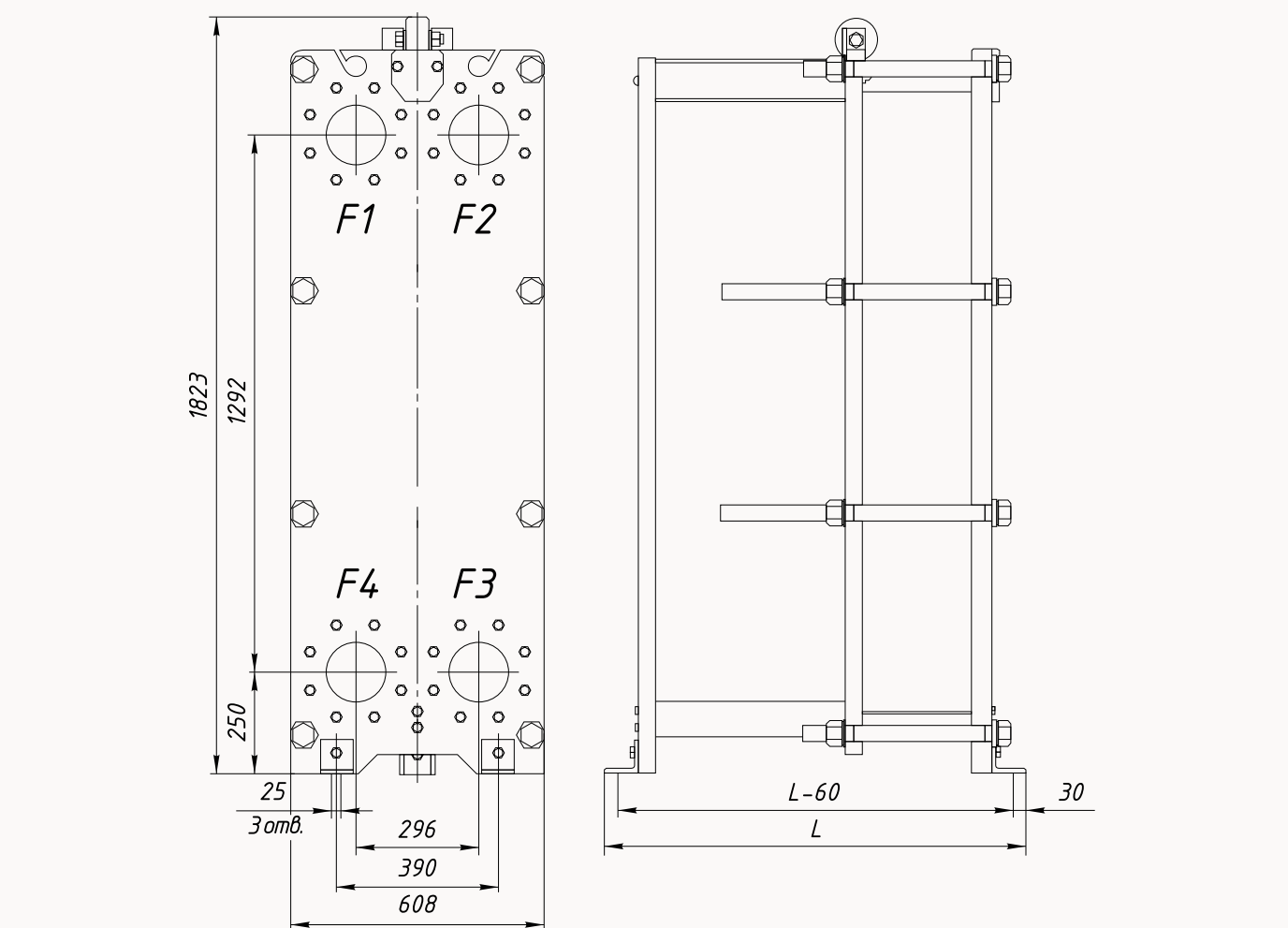
I LP-150M (Расчетное давление 1,0 Мпа)
