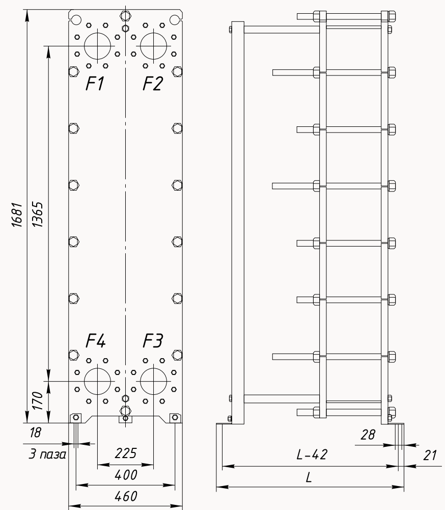
I LP-100M (Расчетное давление 1,0 Мпа)
