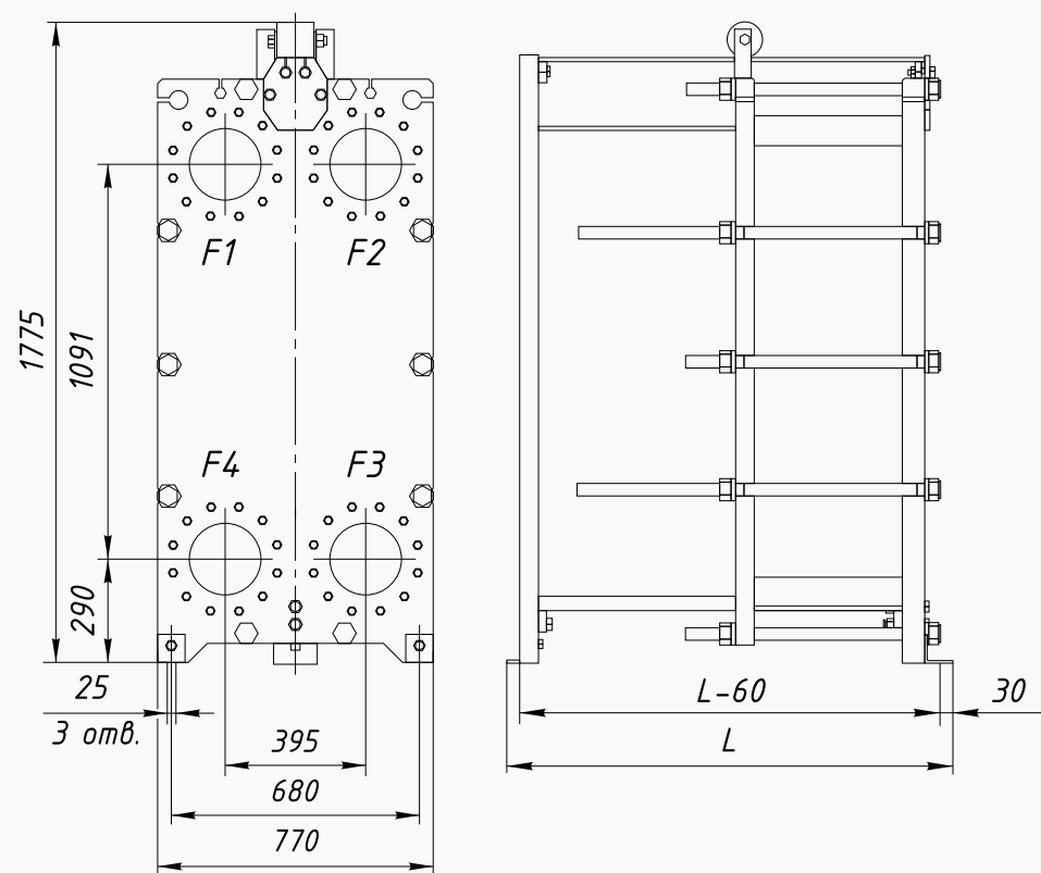
I LP-200M (Расчетное давление 1,0 Мпа)
