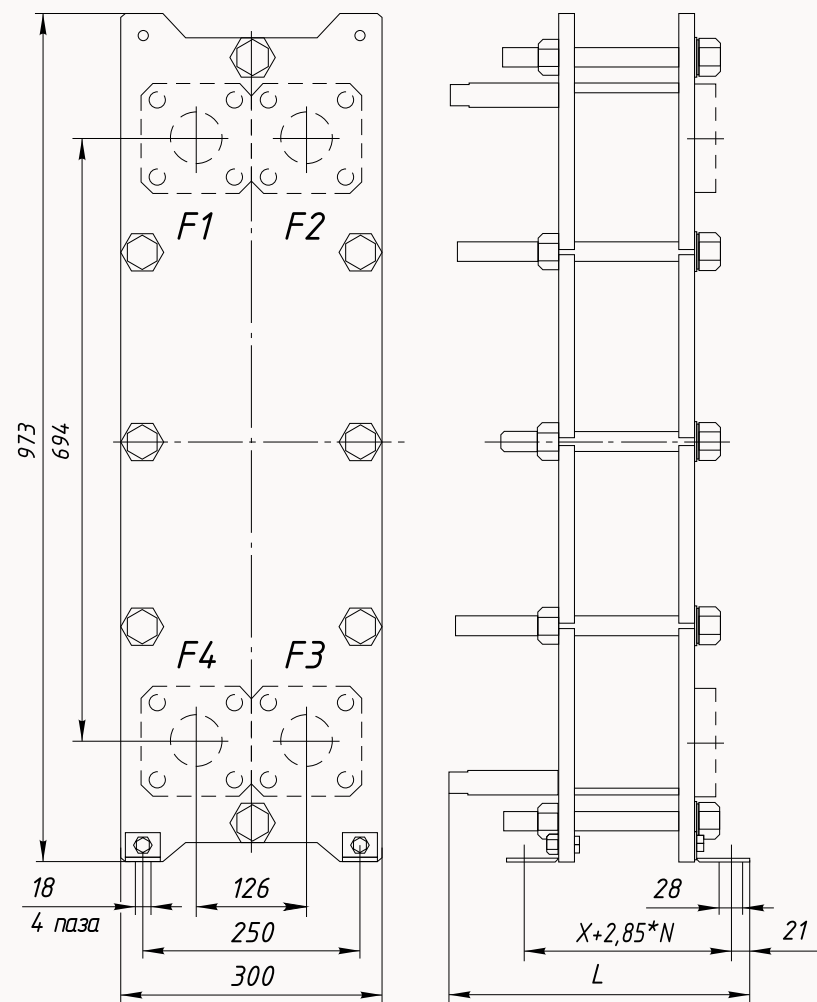
I LP-50M (Расчетное давление 1,0 Мпа)
