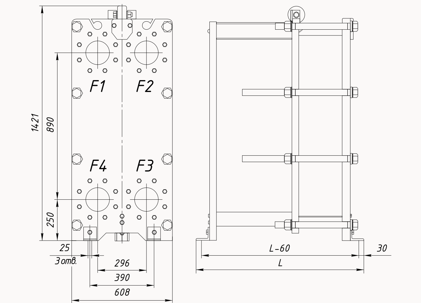
I LP-150S (Расчетное давление 1,0 Мпа)
