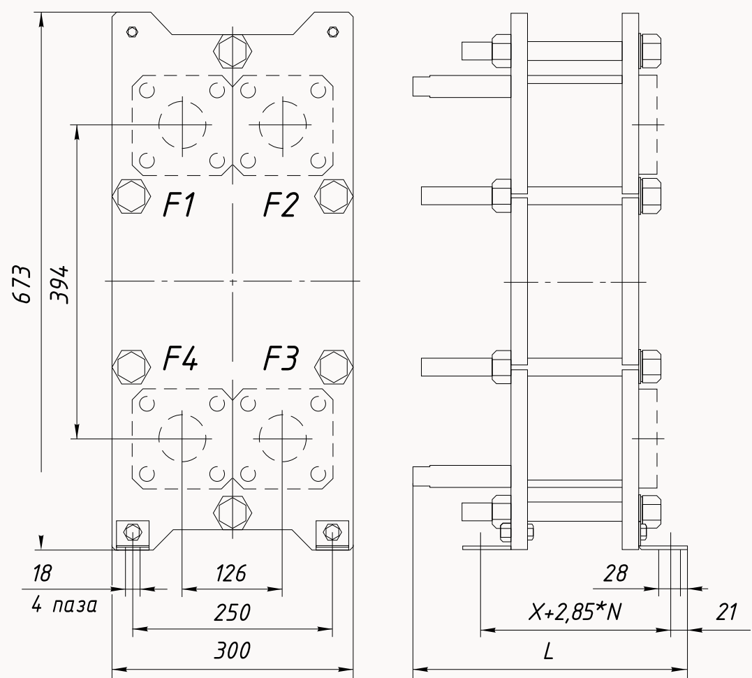
I LP-50S (Расчетное давление 1,0 Мпа)
