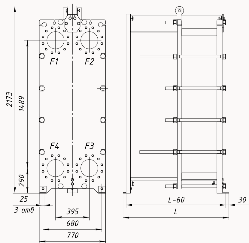
I LP-200L (Расчетное давление 1,0 Мпа)
