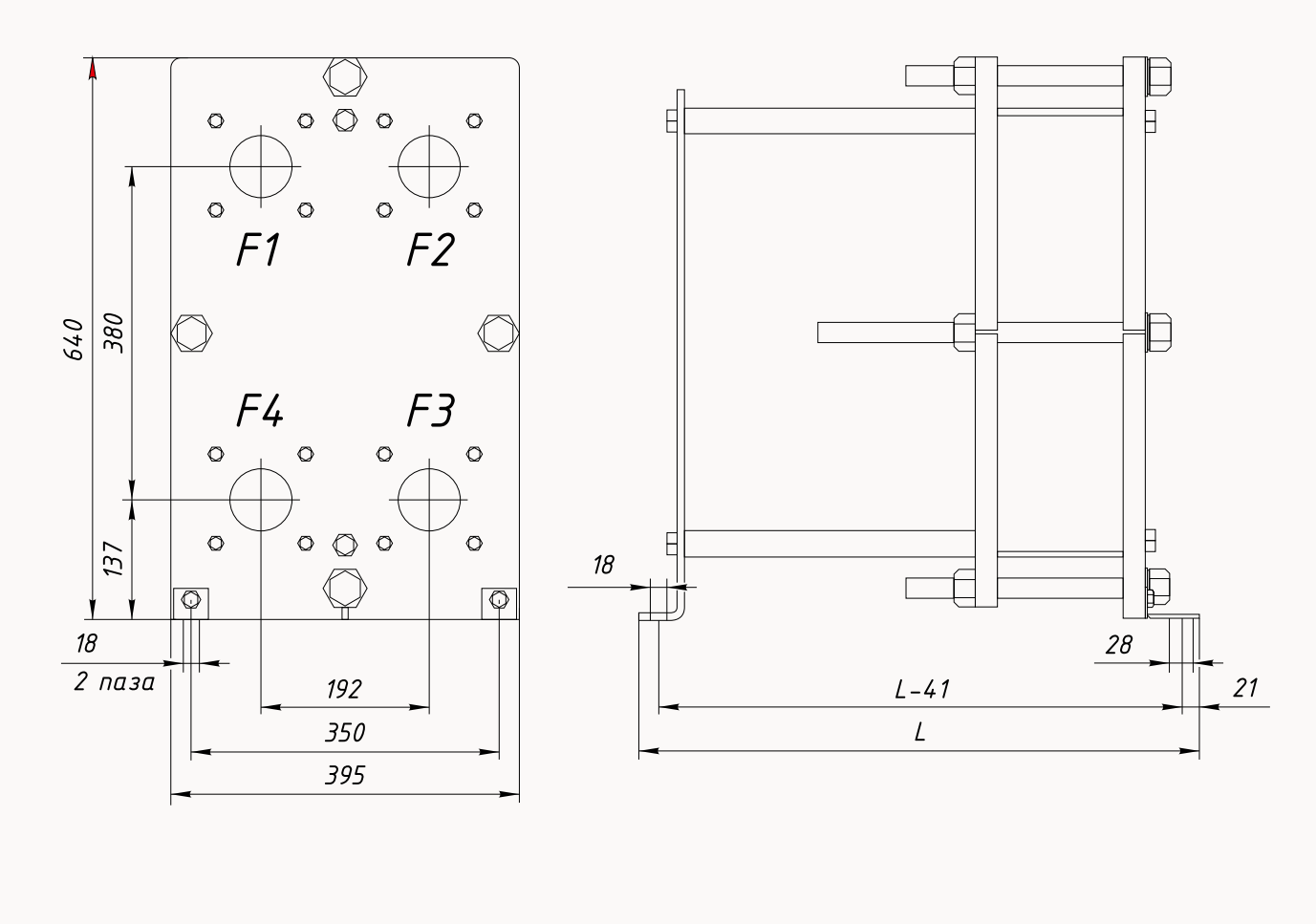
I LP-65S (Расчетное давление 1,0 Мпа)
