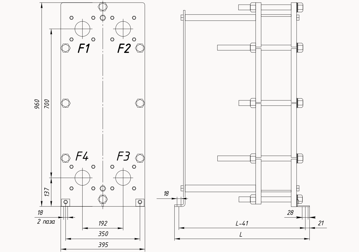
I LP-65M (Расчетное давление 1,0 Мпа)
