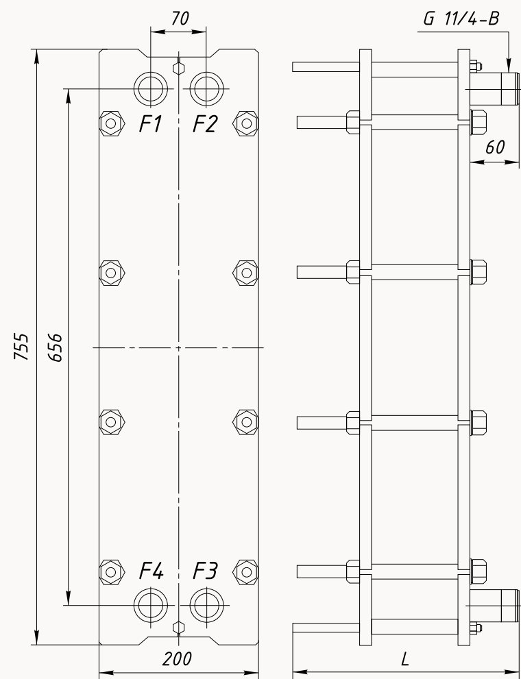
I LP-32M (Расчетное давление 1,0 Мпа)
